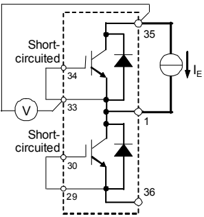
UP / UN IGBT
