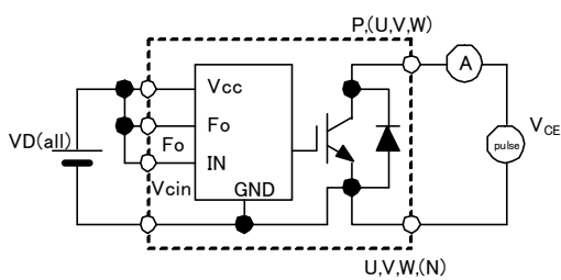
Fig. 5 I_{CES} Test
